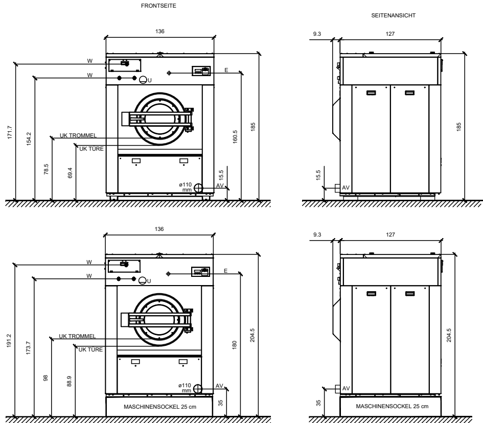
Macchina a carica frontale maxLine 45E
